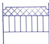
ref.: H-27/1 cabecero rombos de 150 dim.: 160 x 4 x 133
